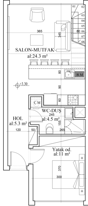
1. KAT
